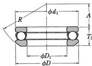
調心球面型
