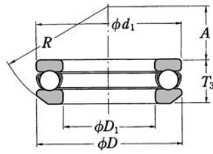
調心球面型
