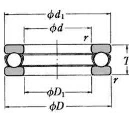
平面座型
