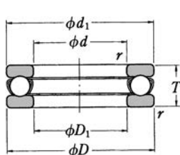
平面座型
