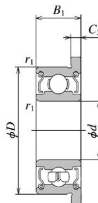
防塵蓋型 Shielded type ZZ · ZZ1
